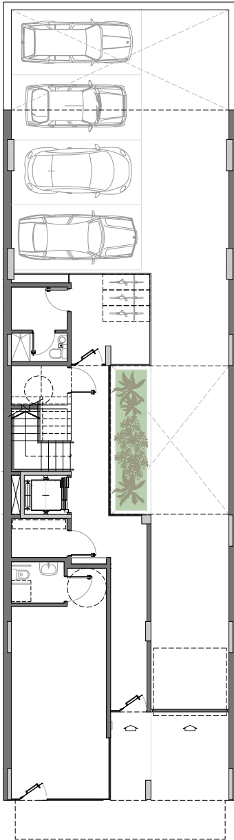
Planta Baja
